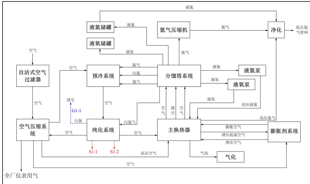
图 4.1-5 空分装置生产工艺流程图
