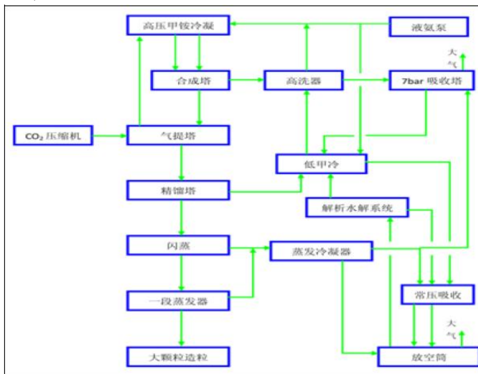
图 4.1-4 尿素生产工艺流程图
