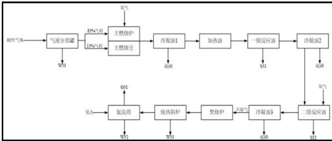
图 4.1-8 硫回收生产工艺流程
