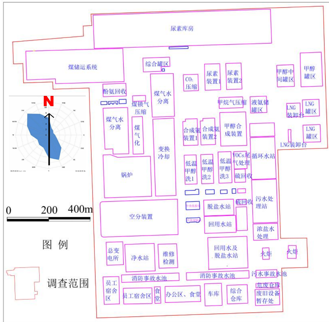
图 4.2-1 厂区平面布置图
