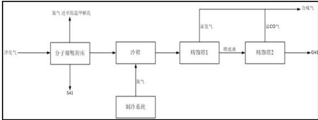
图 4.1-7 甲烷深冷分离生产工艺流程图
