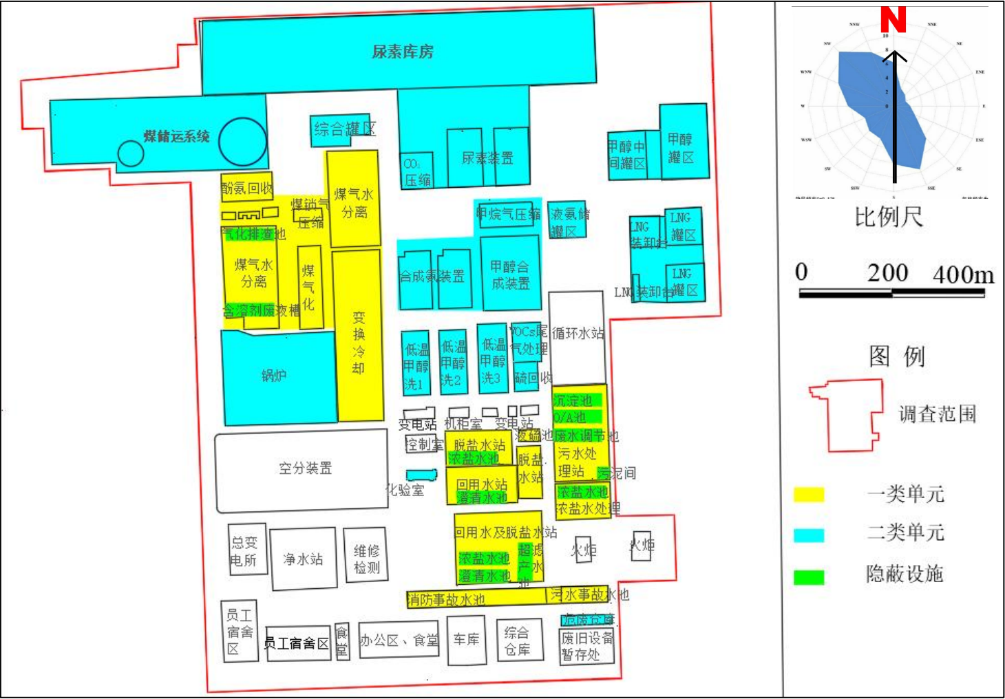
图 4.4-1 重点监测单元平面分布图
