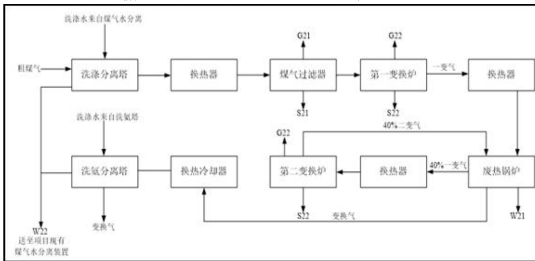
图 4.1-6 变换装置生产工艺流程图
