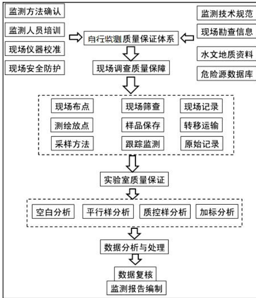
图 8.1-1 土壤自行监测与实验室控制质量保证体系
