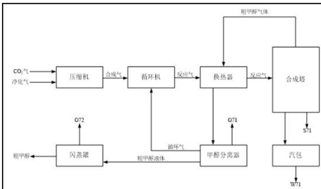
图 4.1-10 甲醇合成生产工艺流程图
