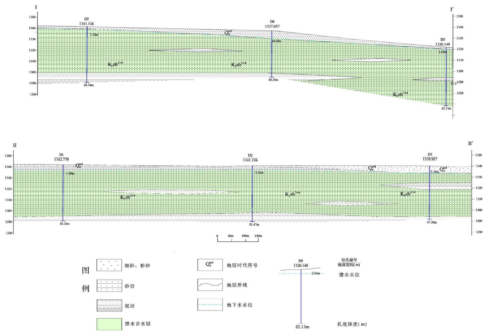
图 3.2-1 水文地质剖面图
