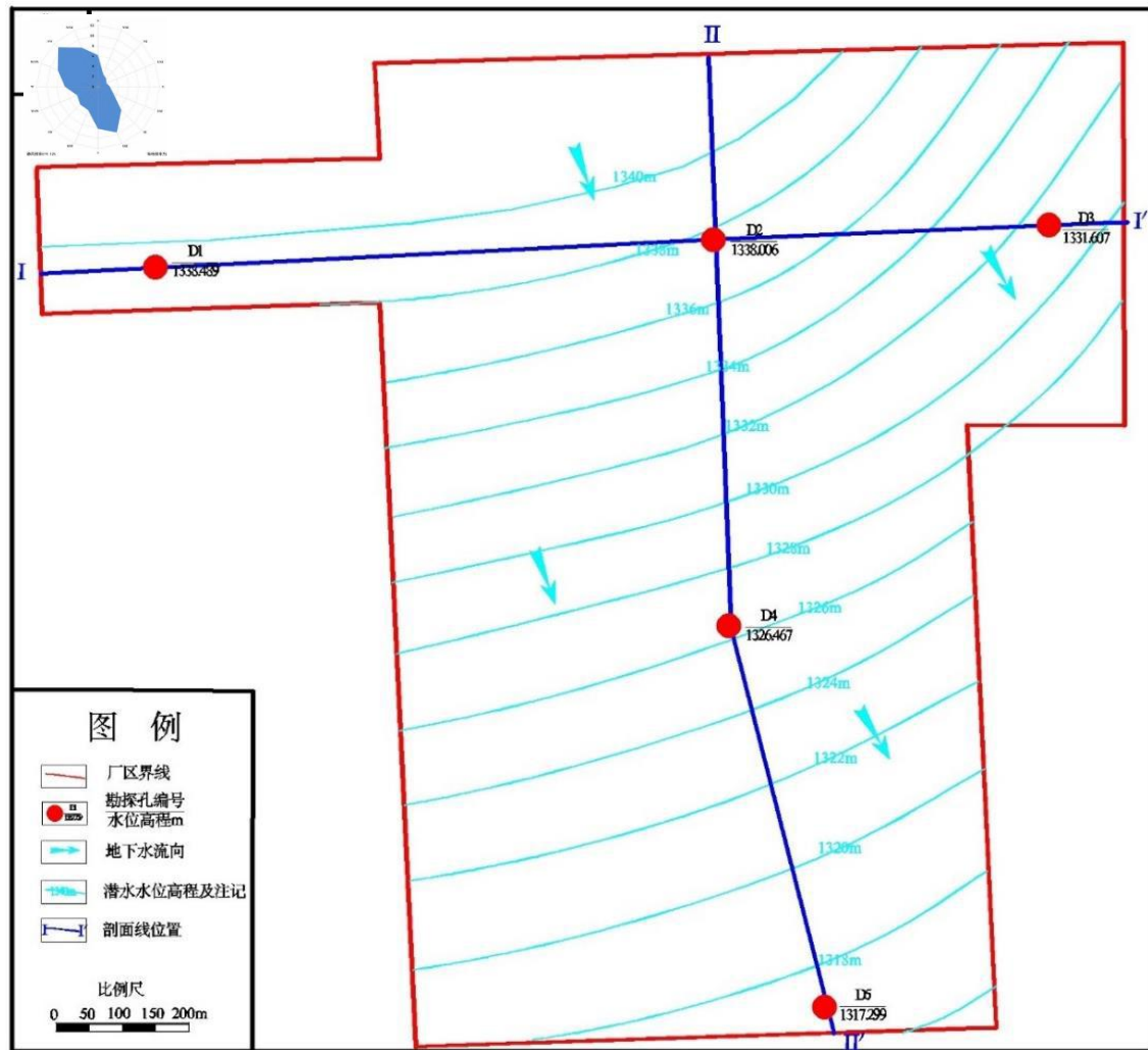
图 3.2-2 潜水水文地质图
