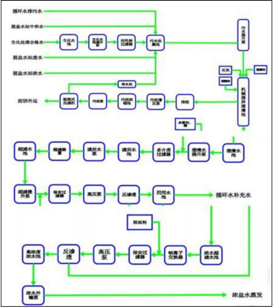
图 4.1-12 回用水站处理系统工艺流程图
