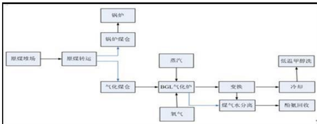
图 4.1-1 气化工艺流程图
