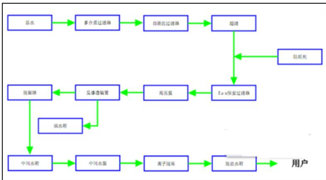
图 4.1-11 脱盐水处理工艺流程
