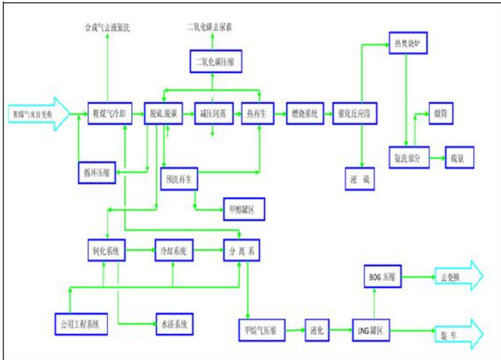
图 4.1-2 净化工艺流程图
