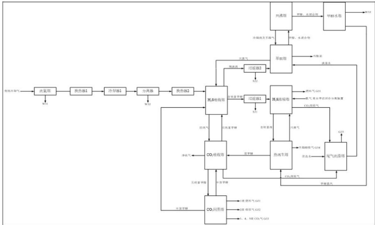
图 4.1-9 低温甲醇洗装置生产工艺流程图
