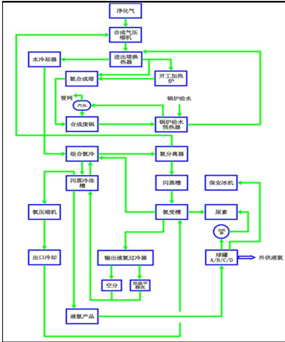
图 4.1-3 合成工艺流程图
